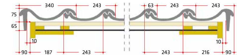
Dachówka skrajna
