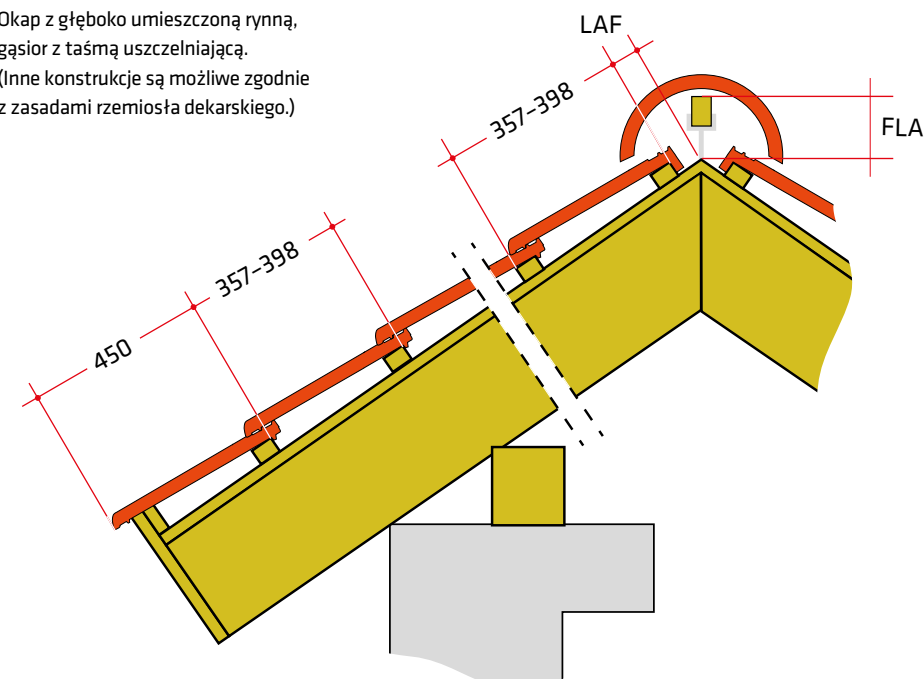
Łaty 30×50 mm
